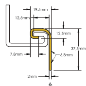
TYPE PW2
